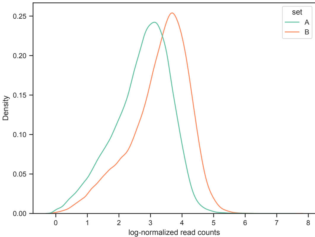
A375_RepA
